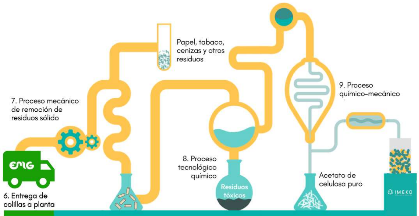
Proceso planta recicladora de colillas.
